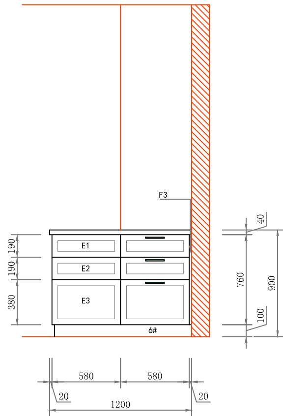
ELEVATION B
