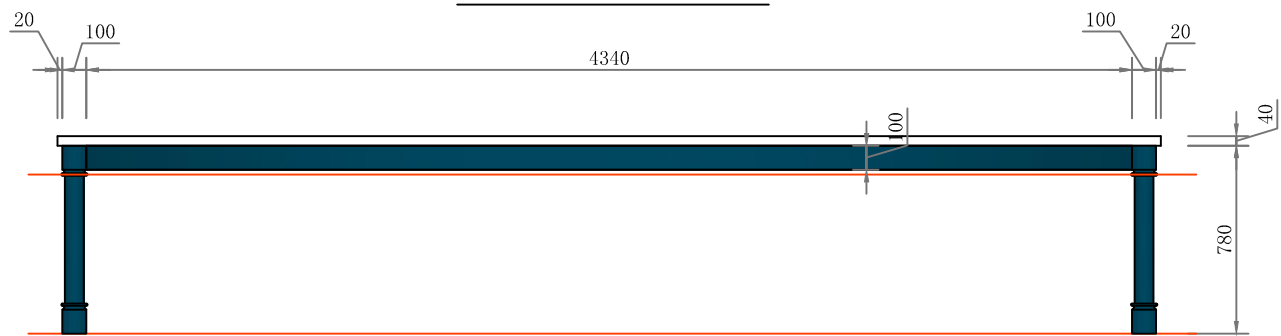
ELEVATION E
