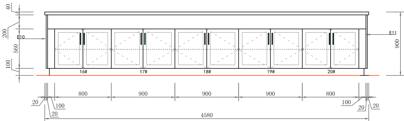
ELEVATION E
