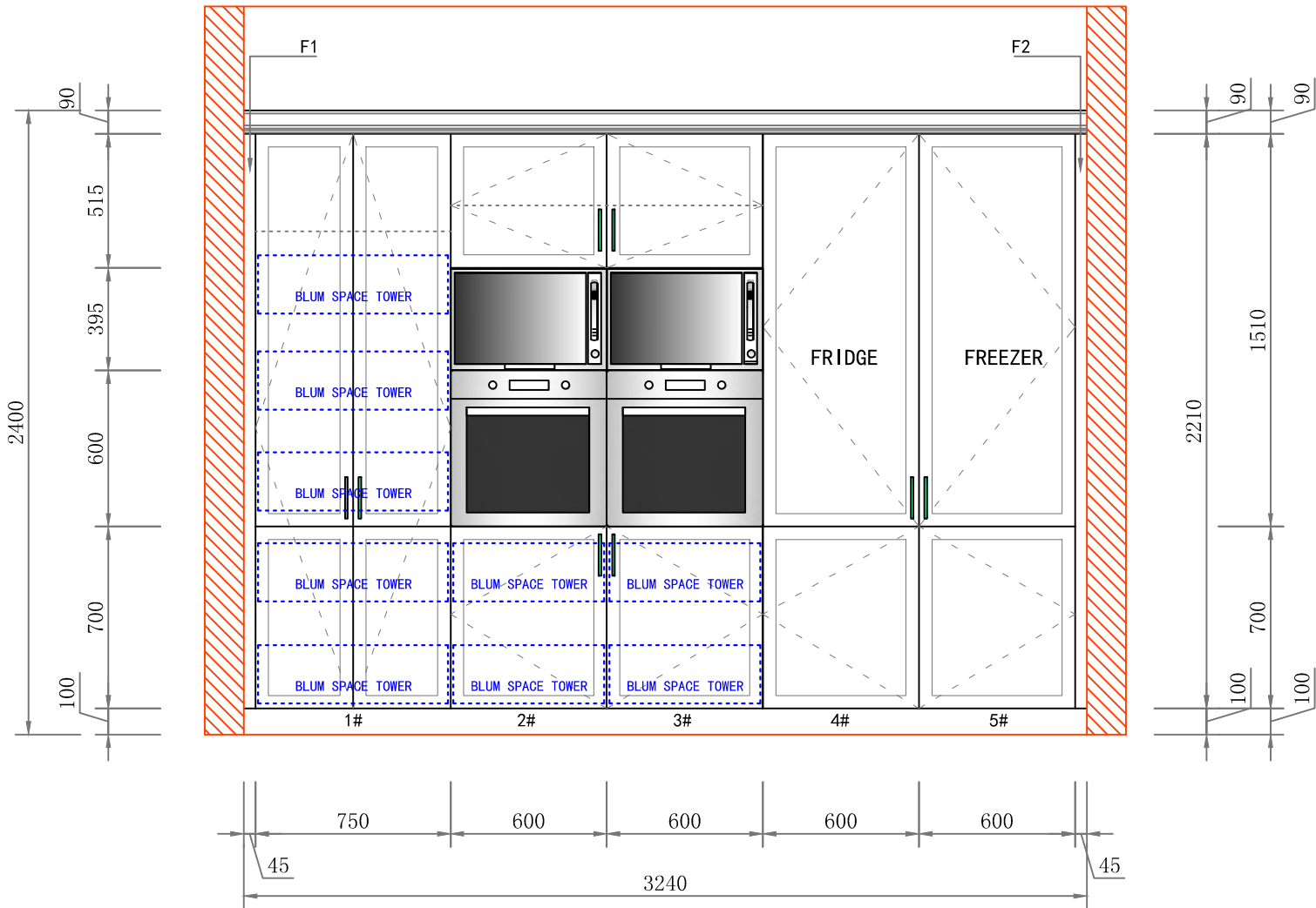
ELEVATION A
