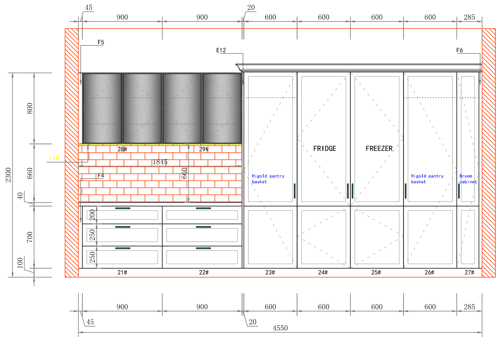
ELEVATION G
