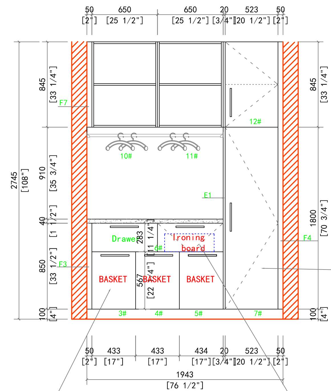
ELEVATION B
