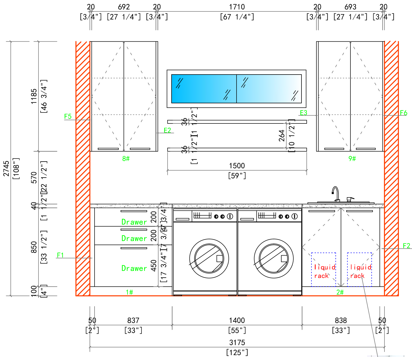
ELEVATION A
