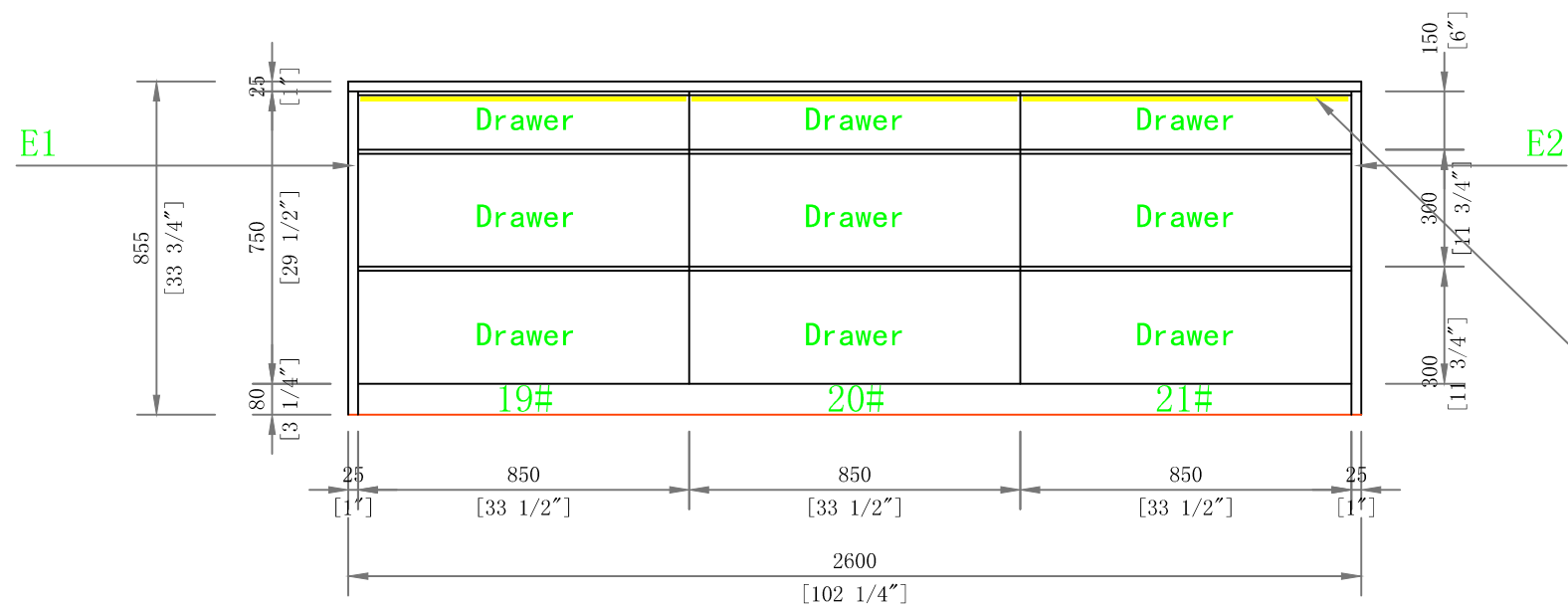
ELEVATION E
