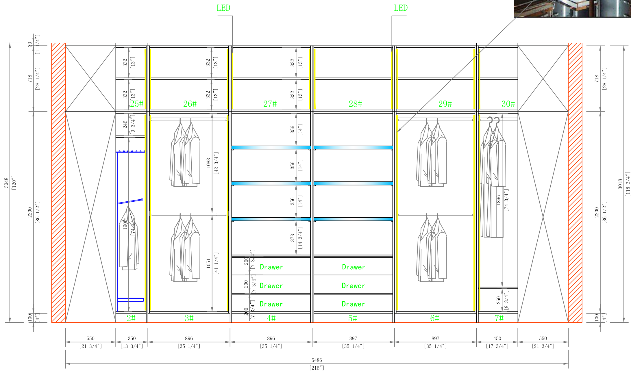
ELEVATION B
