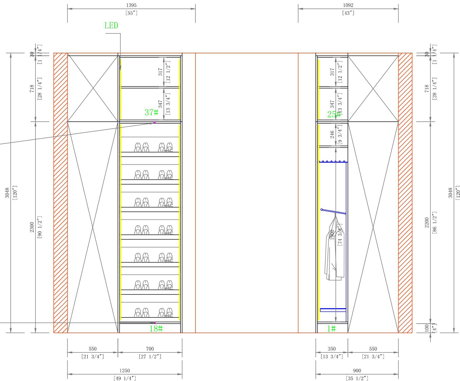
ELEVATION A
