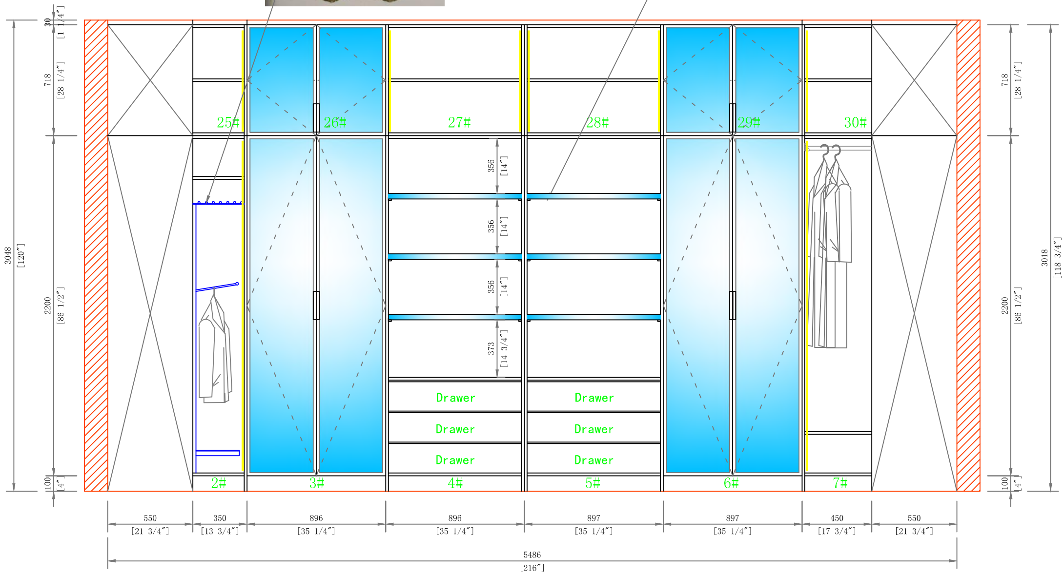
ELEVATION B
