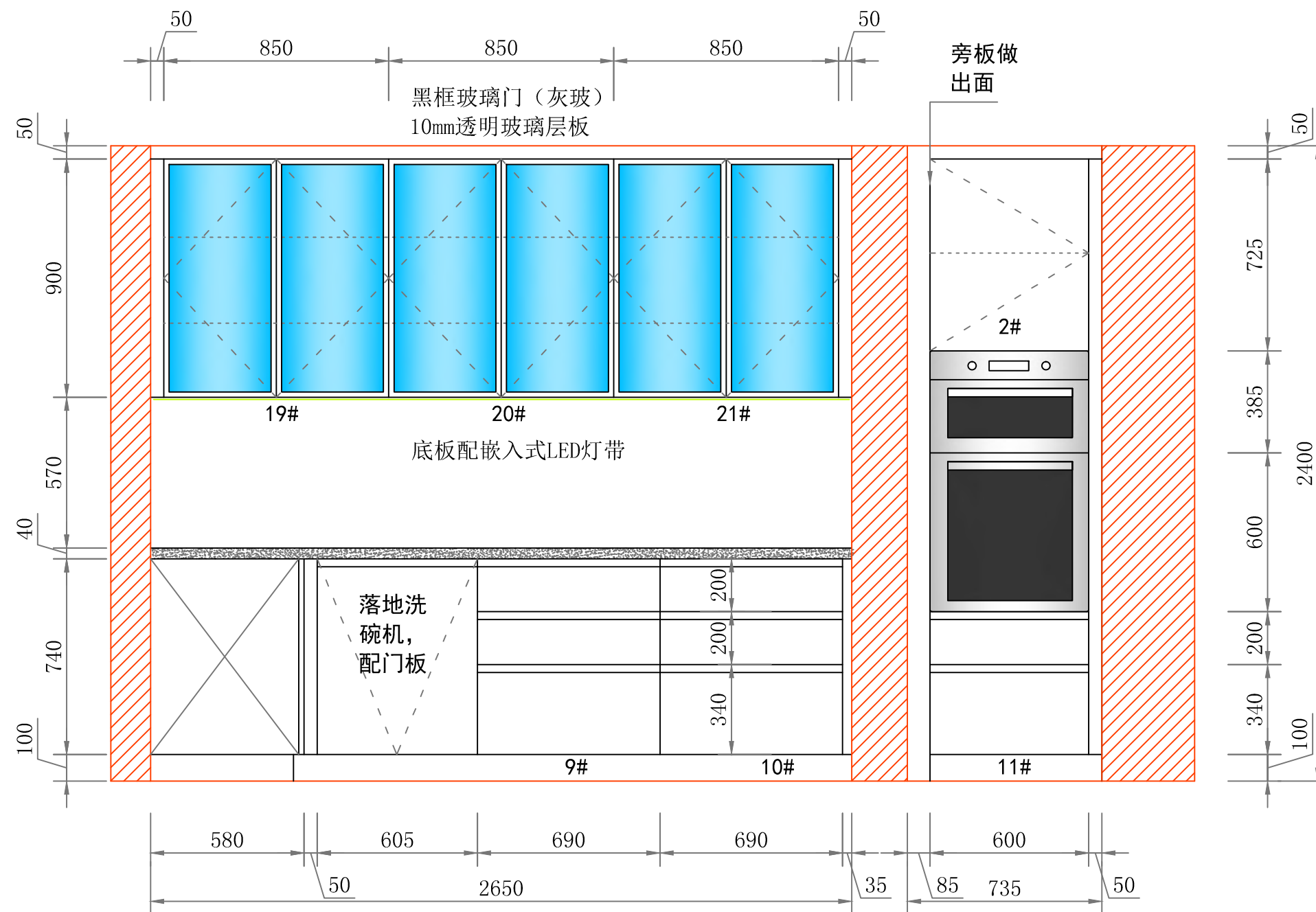
D立面
