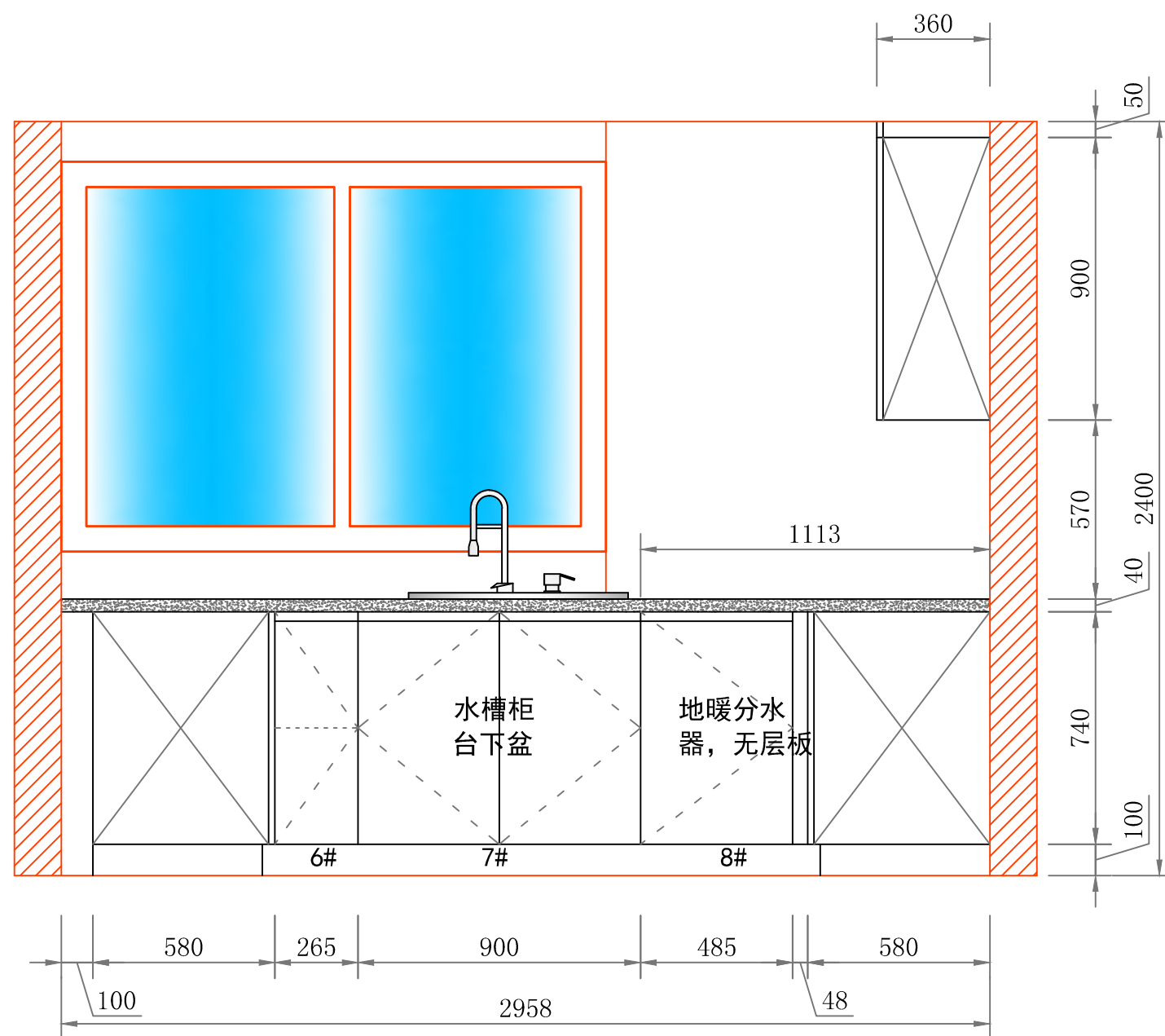
C立面
